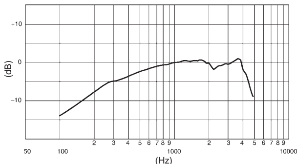
TYPISCHER FREQUENZGANG ABBILDUNG 2
