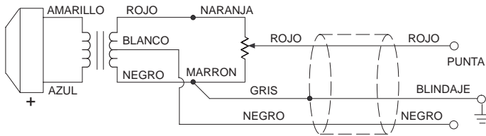
CONEXIONES INTERNAS: SALIDA DE ALTA IMPEDANCIA DESEQUILBRADA
