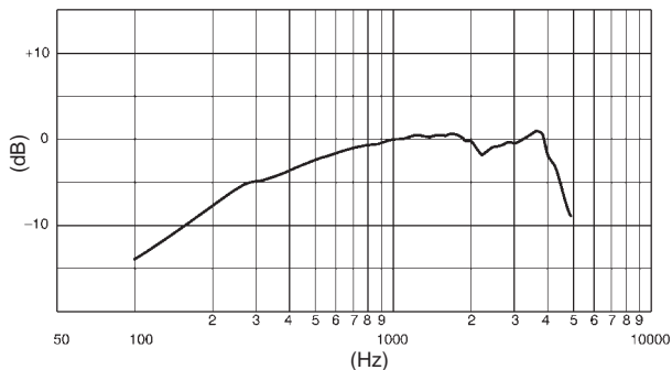
RISPOSTA IN FREQUENZA TIPICA
