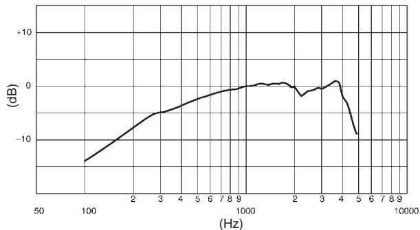
COURBE DE RÉPONSE TYPIQUE FIGURE 2
