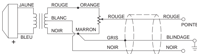
BRANCHEMENTS INTERNES : SORTIE HAUTE IMPÉDANCE ASYMÉTRIQUE
