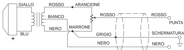
CONNESSIONI INTERNE: USCITA SBILANCIATA AD ALTA IMPEDENZA
